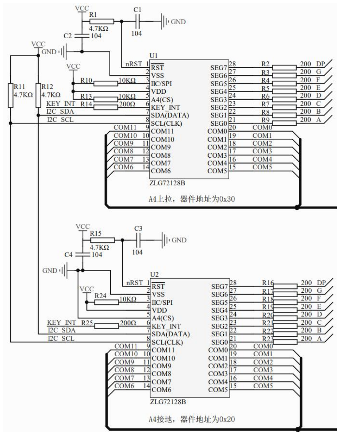
图 5.2 一对 I 2 C 总线挂接两片 ZLG72128B 原理图
