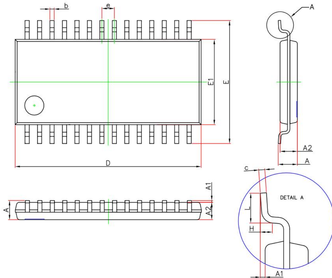
图 7.1 封装尺寸图
