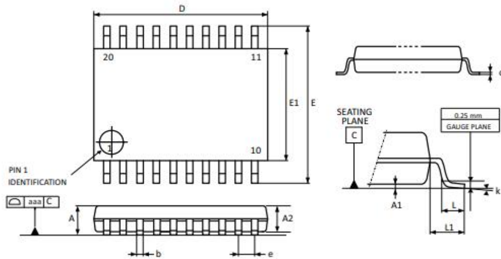
图 6.1 封装尺寸图
