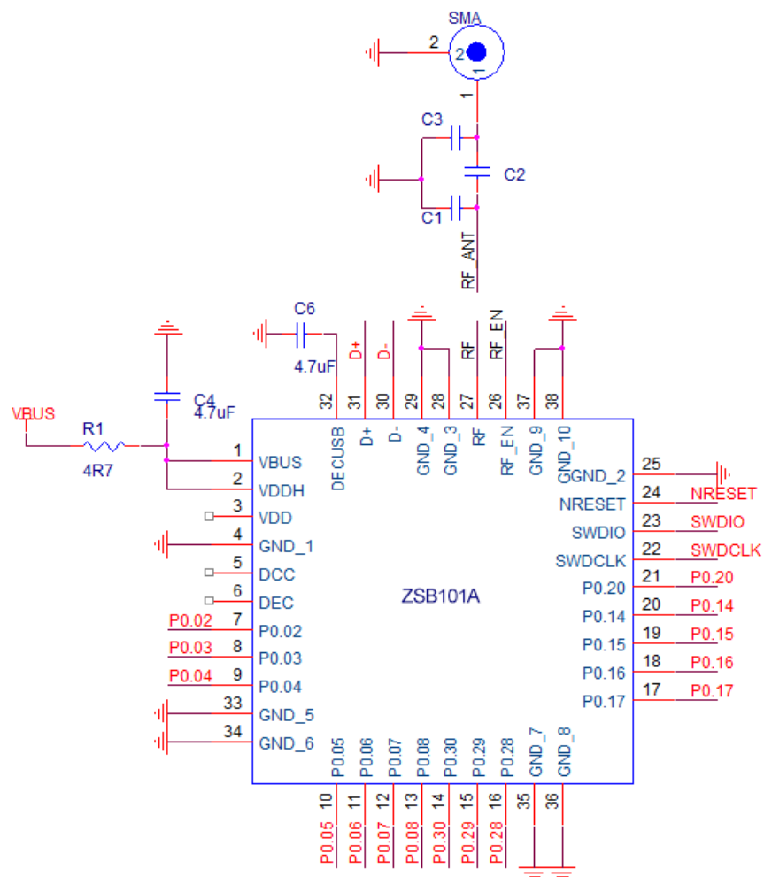
图 5.4 电源配置 d
