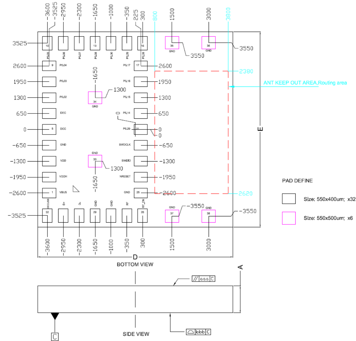
图 6.1 封装尺寸
