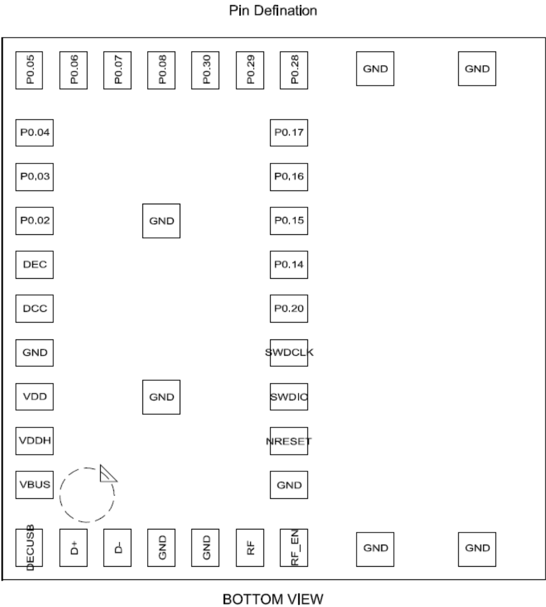
图 2.2 ZSB101A 芯片引脚定义
