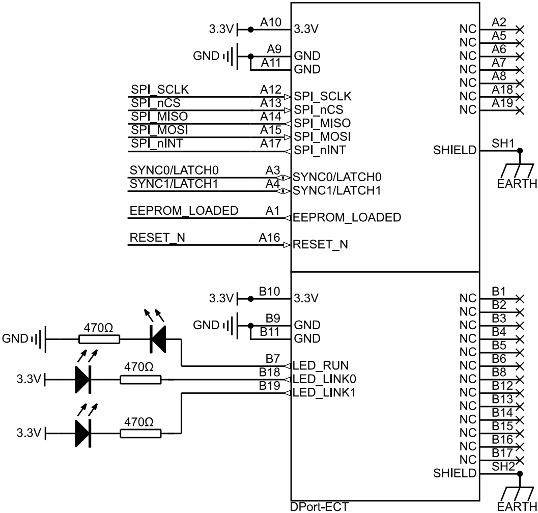
图 3.1 应用电路图
